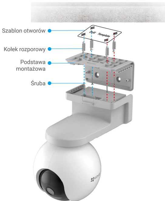
Rys. 1 Montaż sufitowy
