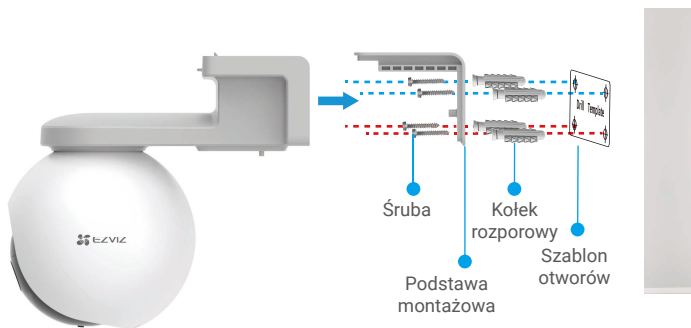
Rys. 2 Montaż ścienny
