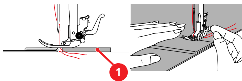
1 Przyrząd kompensacji wysokości materiału
