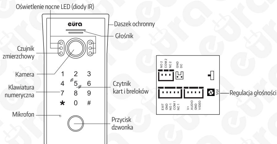
Rys. 1 Budowa kasecy zewnętrznej
