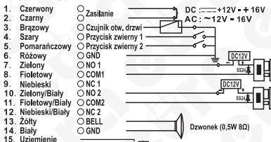
Rys. 6. Schemat połączeń zamków szyfrowych AC-20C7 i AC-30C7
