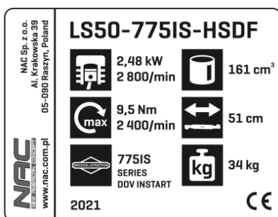
Tabliczka znamionowa
