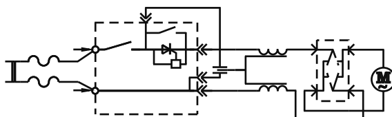
Schemat elektryczny
