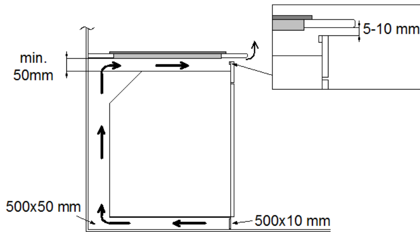
Zabudowa w blacie nad piekarnikiem z wentylacją
