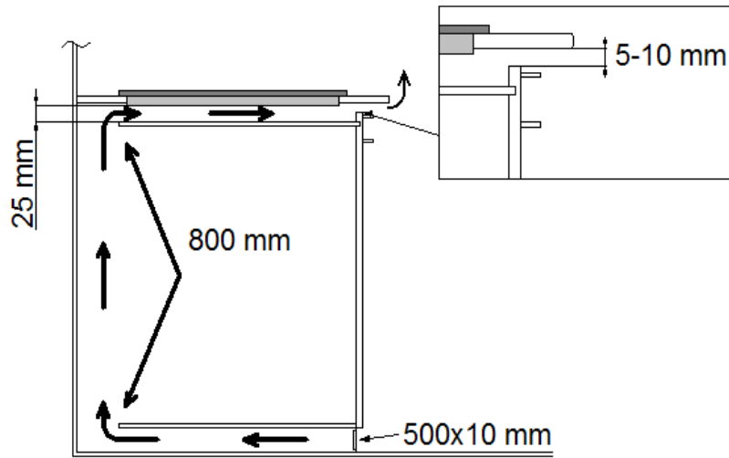
Zabudowa w blacie szafki
